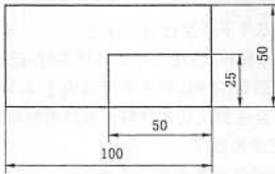
图 8 试样尺寸
